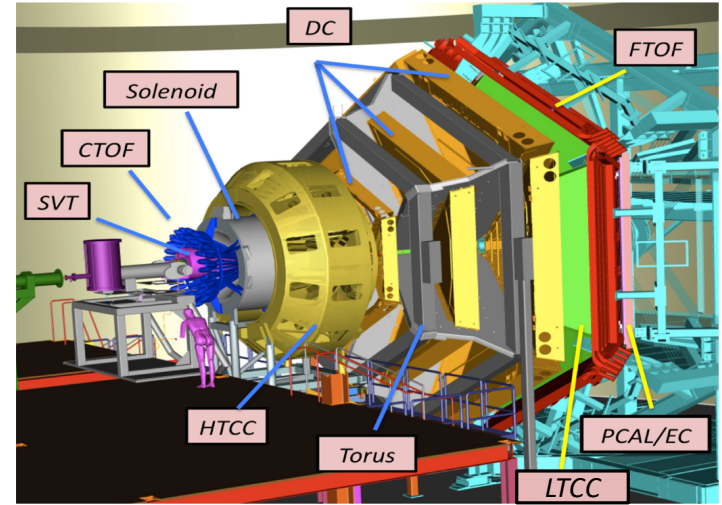
Clas12/Hall B Detector
