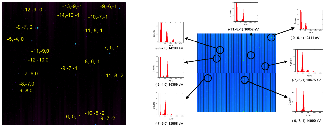
Figure 7 White light microdiffraction at ALS BL 12.3.2 with Berkeley Lab FastCCD.
